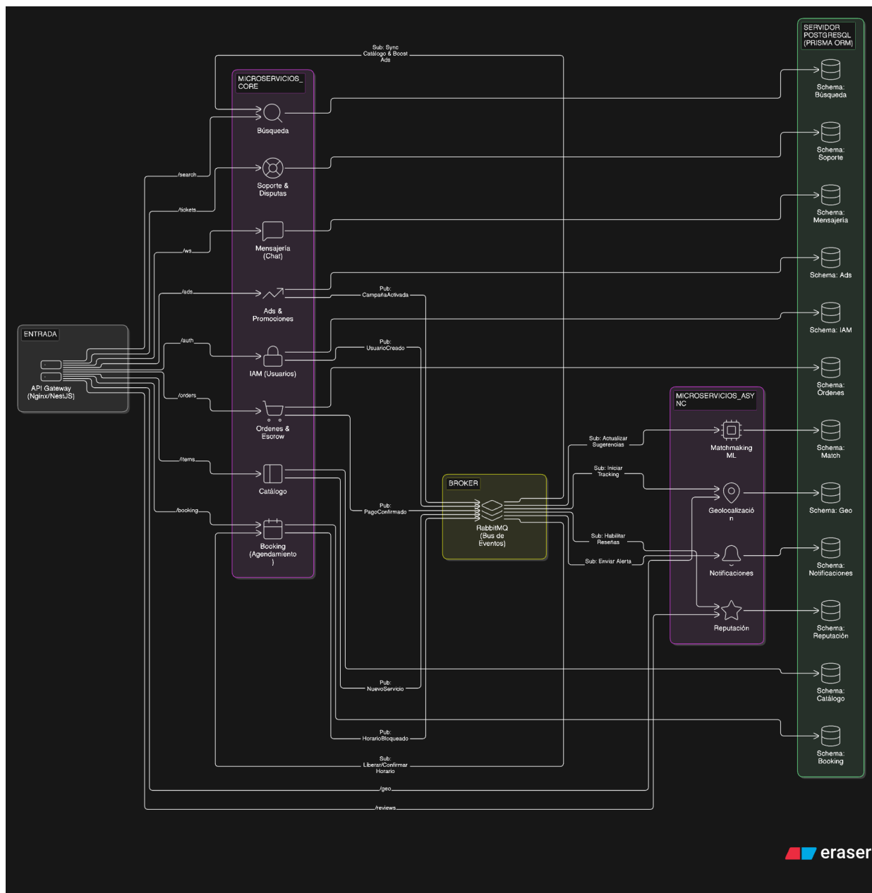
Figura 5: Diagrama de arquitectura de microservicios.
