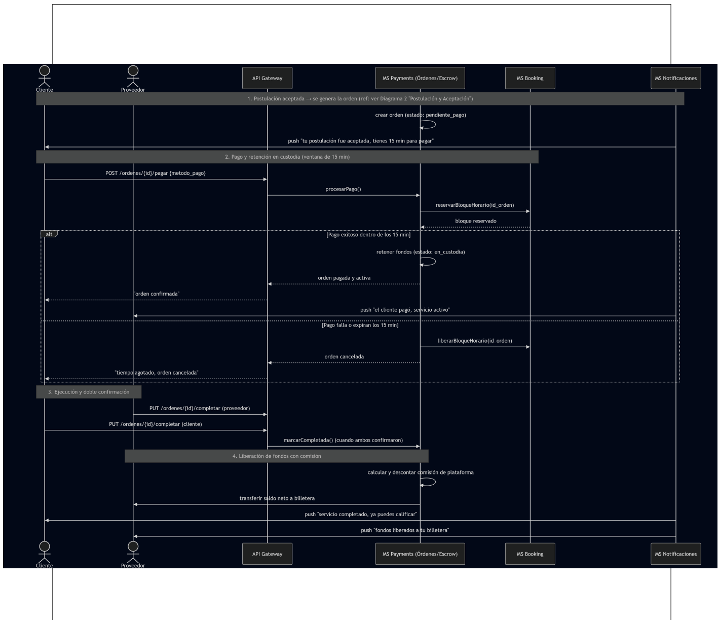
Figura 7: Diagrama de secuencia.
