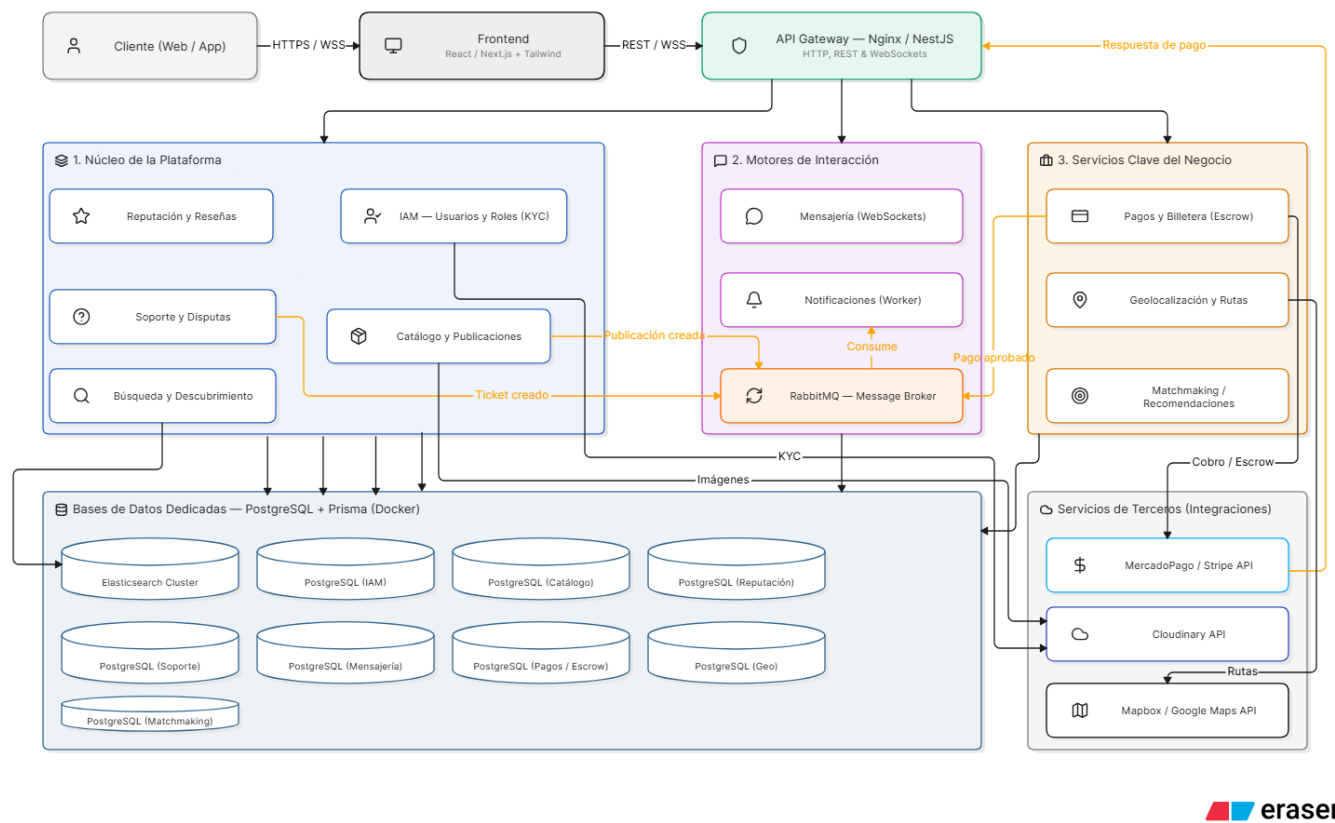
Diagrama de Arquitectura de Software
